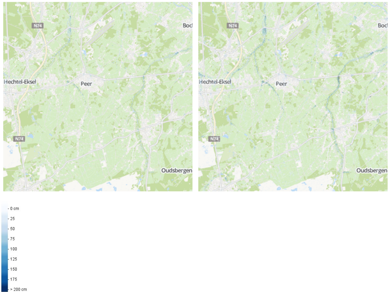
Figuur 17 | Waterdiepte in Peer, in cm (huidig klimaat en 2100)
