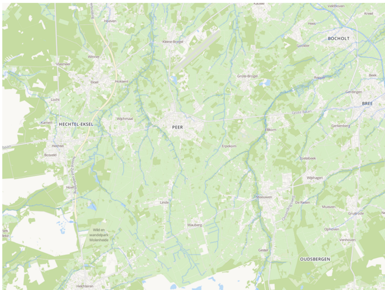
Figuur 13 | Waterlopen in Peer
