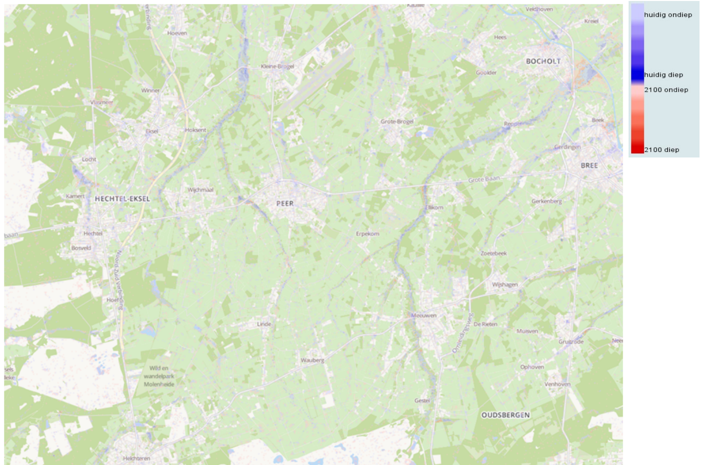
Figuur 18 | Aangroei overstroombaar gebied in Peer (2100)
