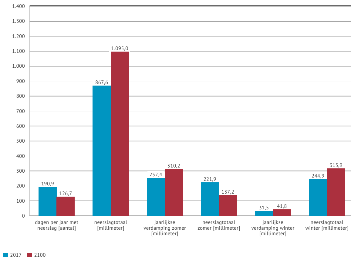
Figuur 24 | Evolutie van de (totale) neerslag en potentiële verdamping in Maasmechelen (huidig klimaat en 2100)
