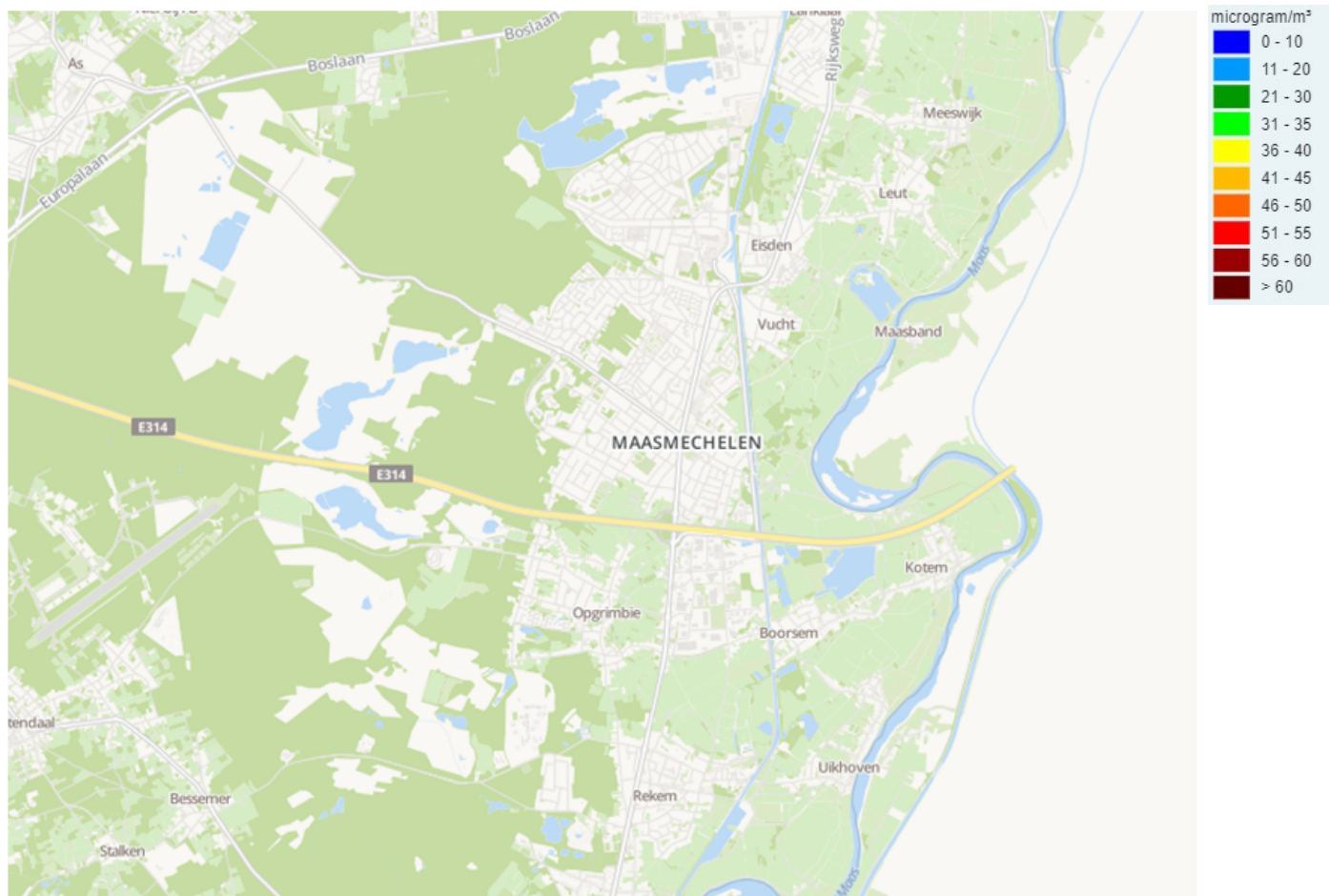
Figuur 09 | Jaargemiddelde ozon (microgram/m 3 ) in Maasmechelen (2017)
