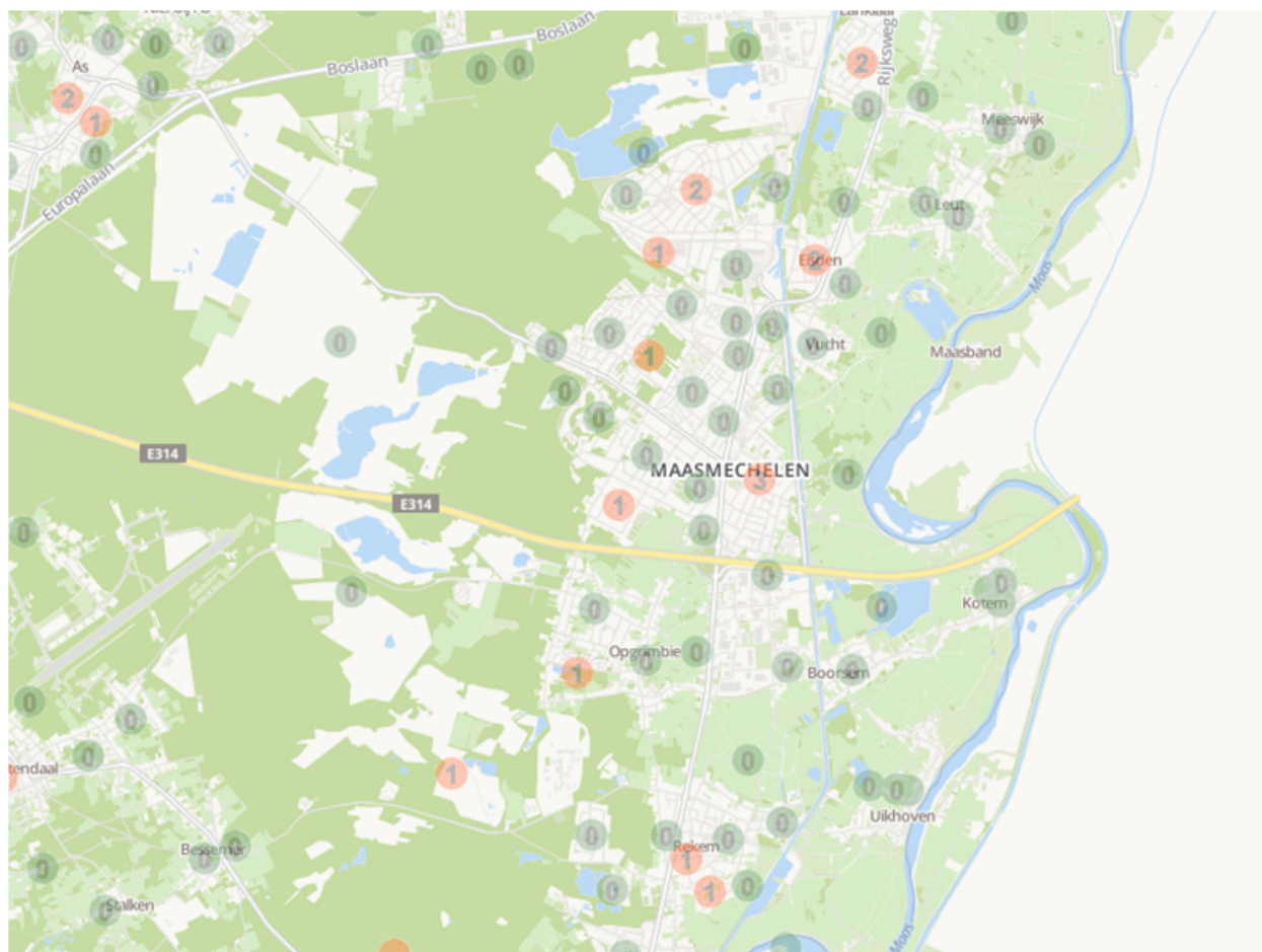
Figuur 21 | Gevaarlijk overstroombare kwetsbare instellingen in Maasmechelen (2100)
