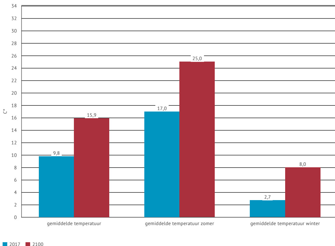
Figuur 32 | Gemiddelde temperatuur in Maasmechelen (huidig klimaat en 2100)
