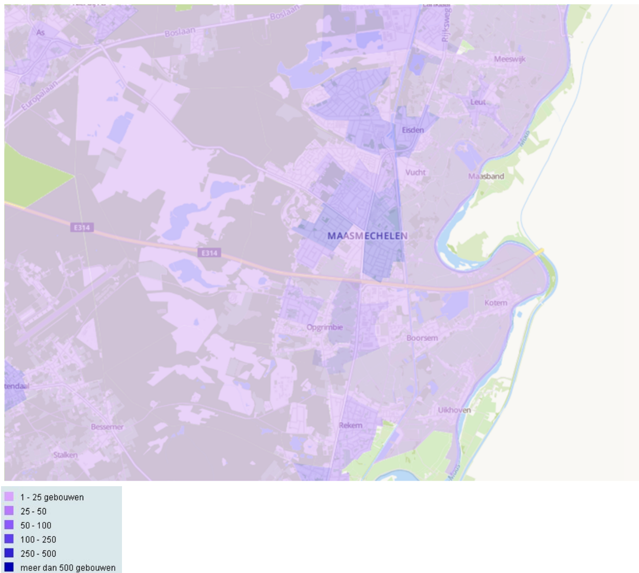
Figuur 22 | Aantal gevaarlijk overstroombare gebouwen in Maasmechelen (2100)
