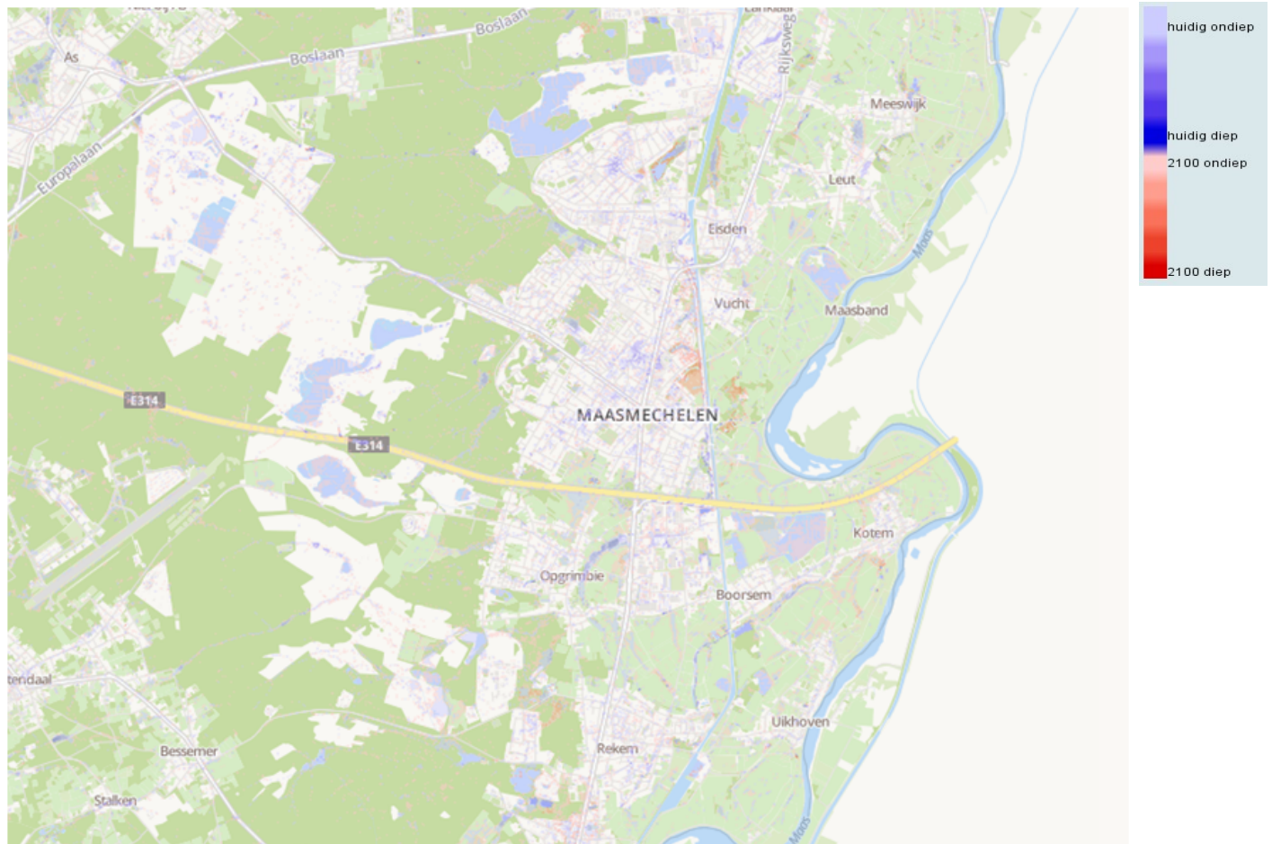
Figuur 18 | Aangroei overstroombaar gebied in Maasmechelen (2100)
