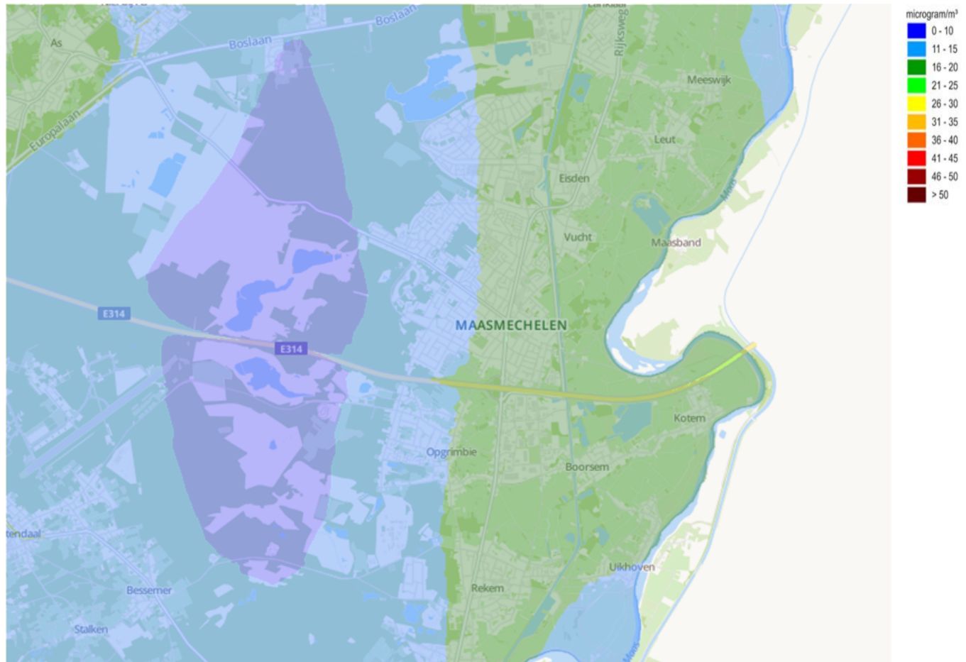
Figuur 42 | Fijn stof in Maasmechelen (2017)
