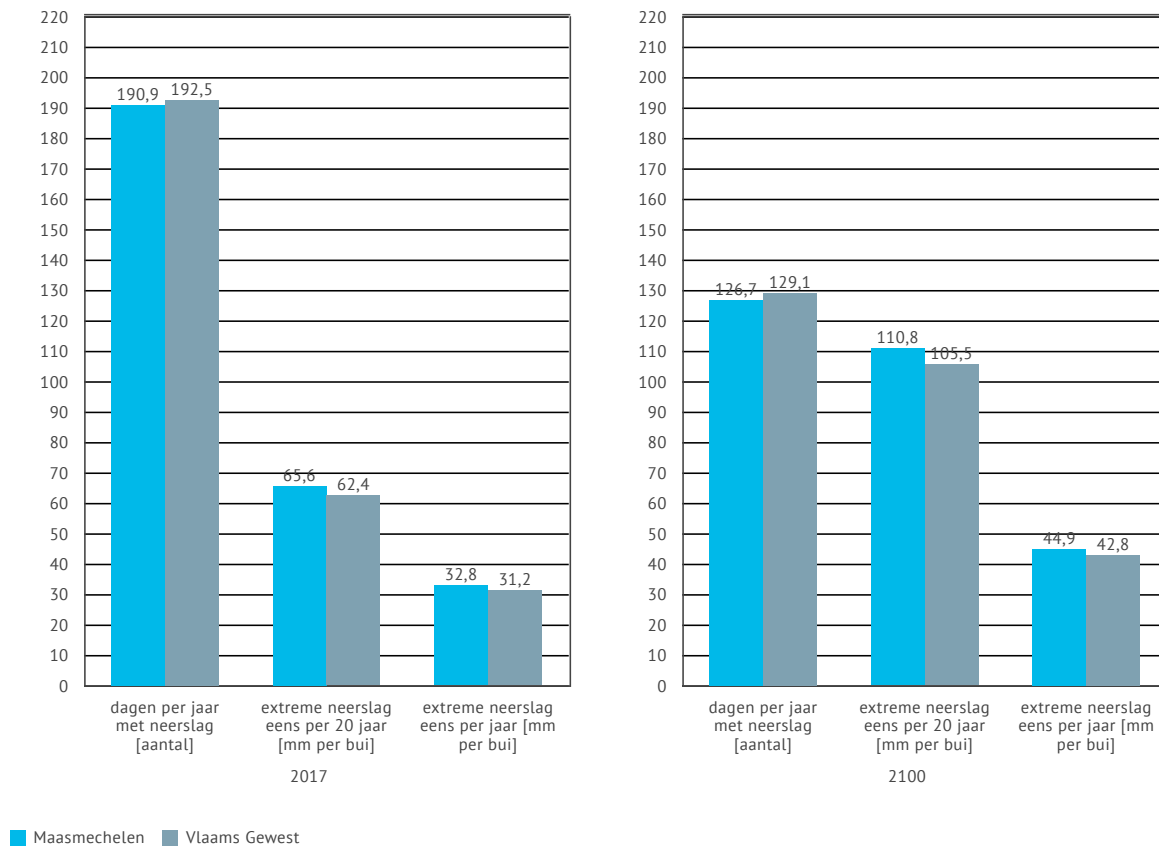
Figuur 12 | Evolutie van (extreme) neerslag in Maasmechelen (huidig klimaat en 2100)
