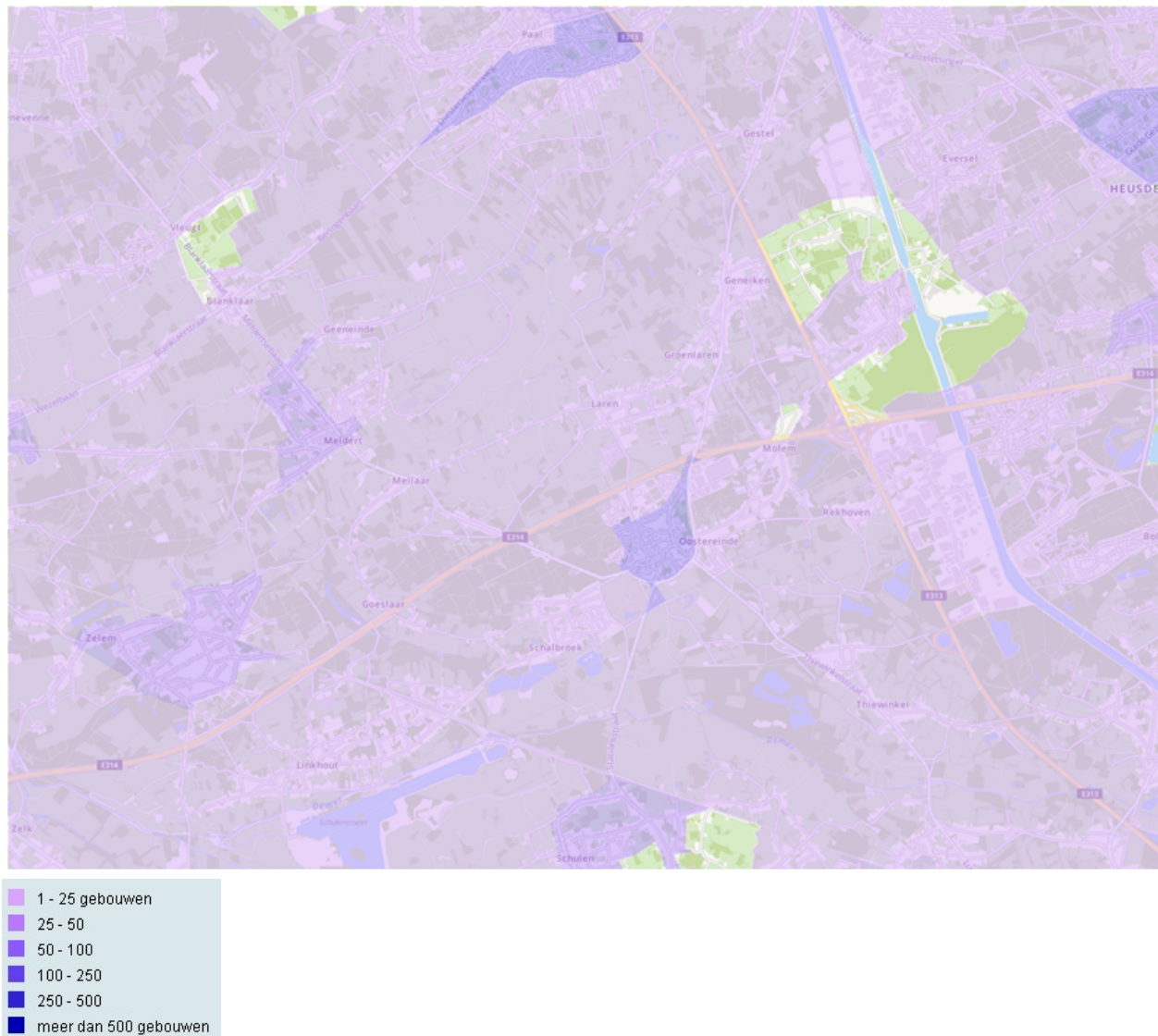
Figuur 22 | Aantal gevaarlijk overstroombare gebouwen in Lummen (2100)
