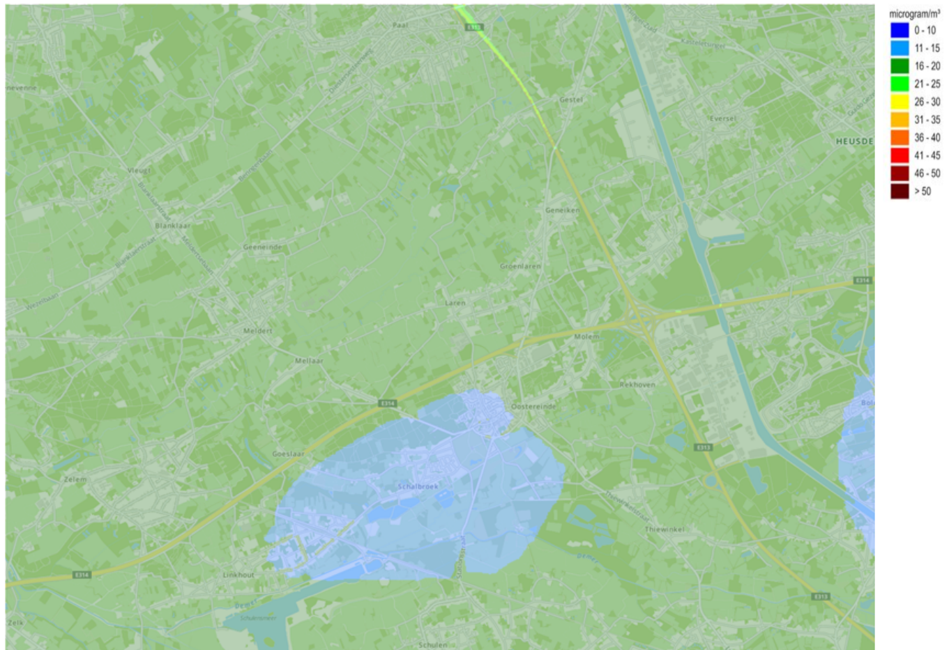
Figuur 42 | Fijn stof in Lummen (2017)
