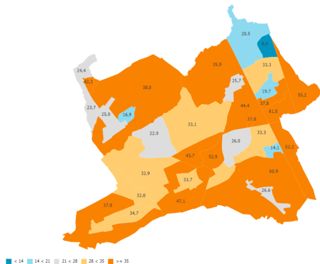
Figuur 35 | Grijsdruk per statistische sector in Lummen (2018)
