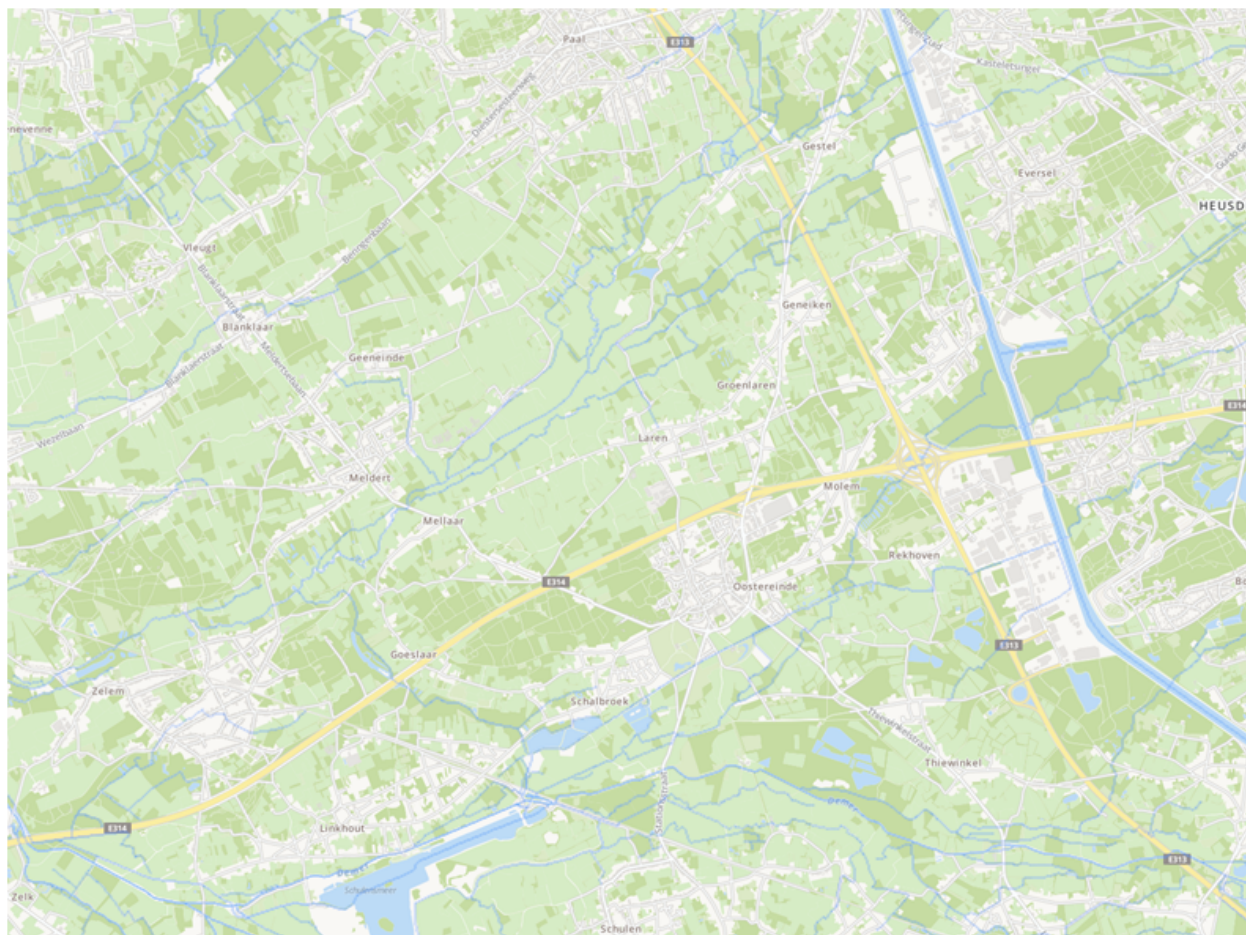
Figuur 13 | Waterlopen in Lummen
