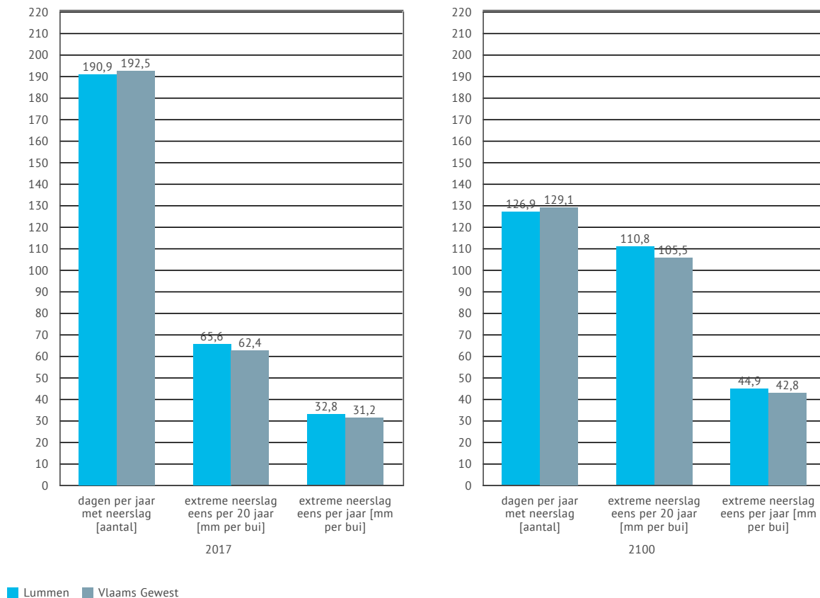
Figuur 12 | Evolutie van (extreme) neerslag in Lummen (huidig klimaat en 2100)
