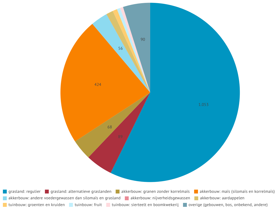
Figuur 38 | Overzicht van de teelten in hectare in Lummen (2018)
