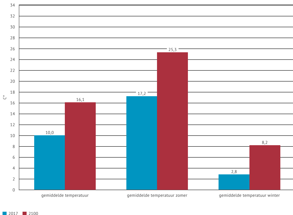
Figuur 32 | Gemiddelde temperatuur in Lummen (huidig klimaat en 2100)
