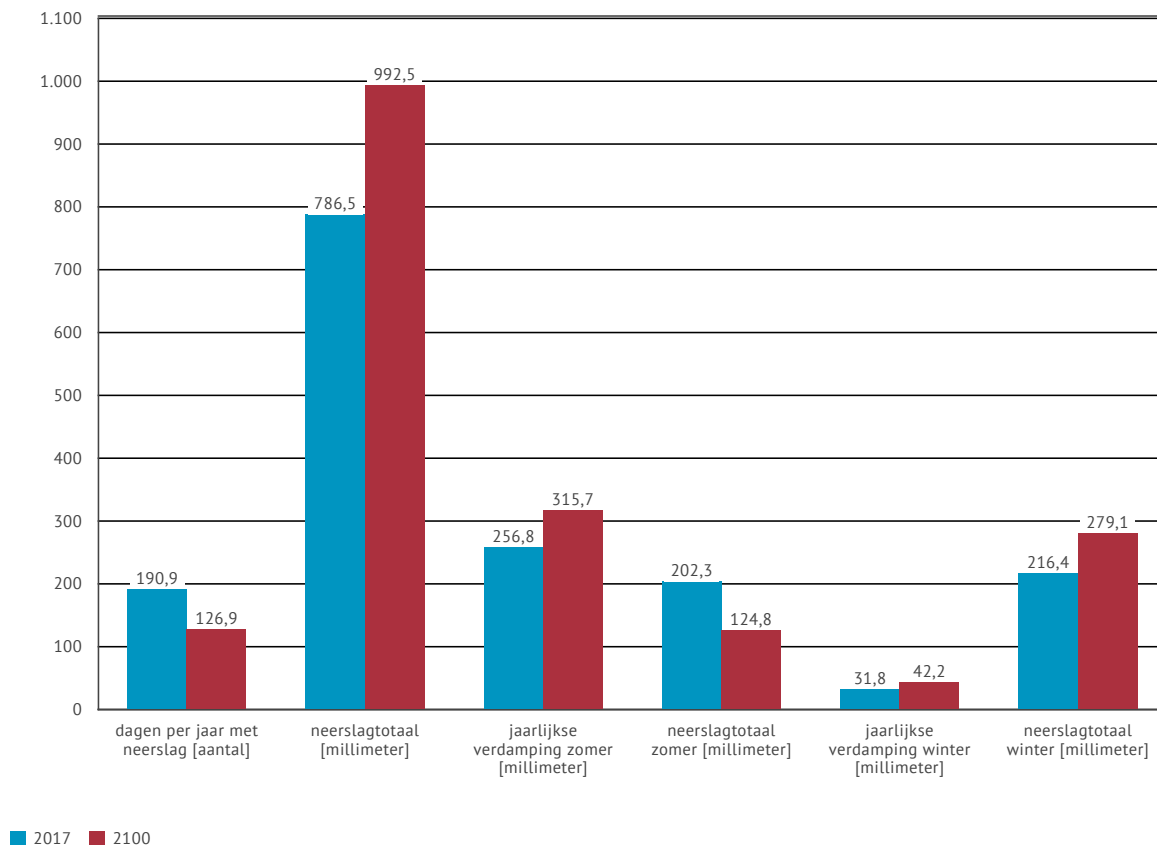
Figuur 24 | Evolutie van de (totale) neerslag en potentiële verdamping in Lummen (huidig klimaat en 2100)
