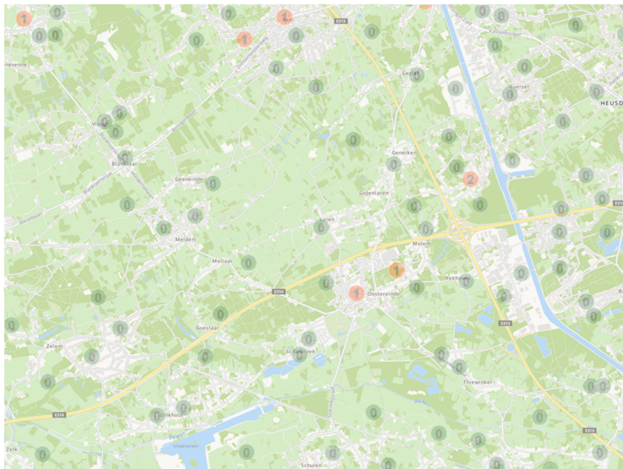
Figuur 21 | Gevaarlijk overstroombare kwetsbare instellingen in Lummen (2100)
