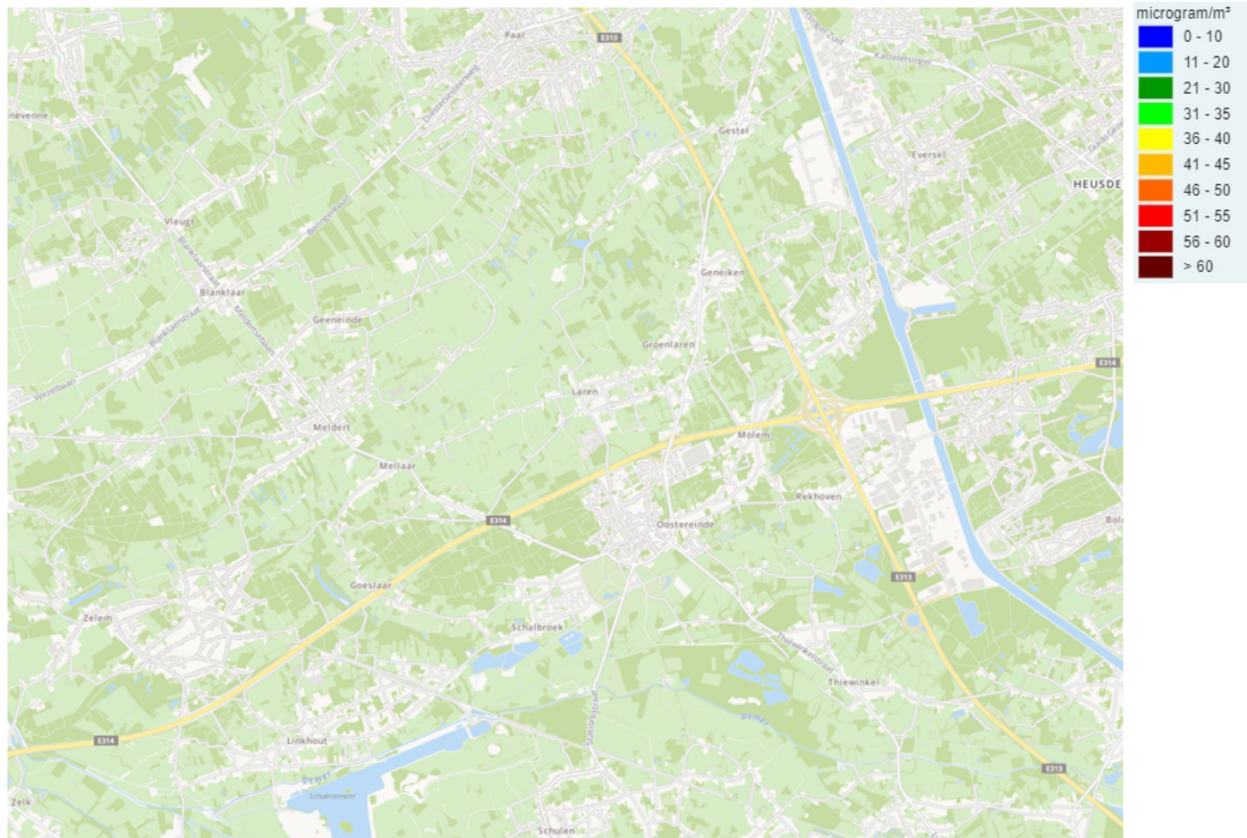
Figuur 09 | Jaargemiddelde ozon (microgram/m 3 ) in Lummen (2017)
