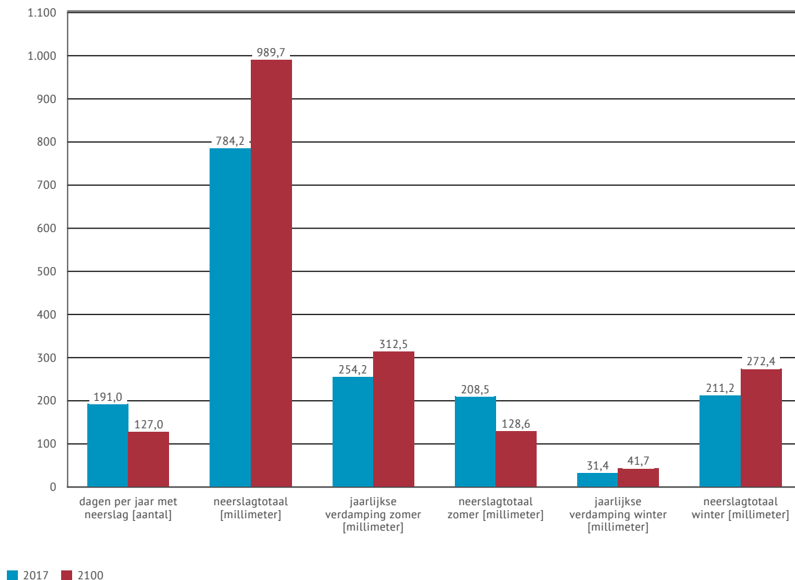
Figuur 24 | Evolutie van de (totale) neerslag en potentiële verdamping in Kortesse (huidig klimaat en 2100)
