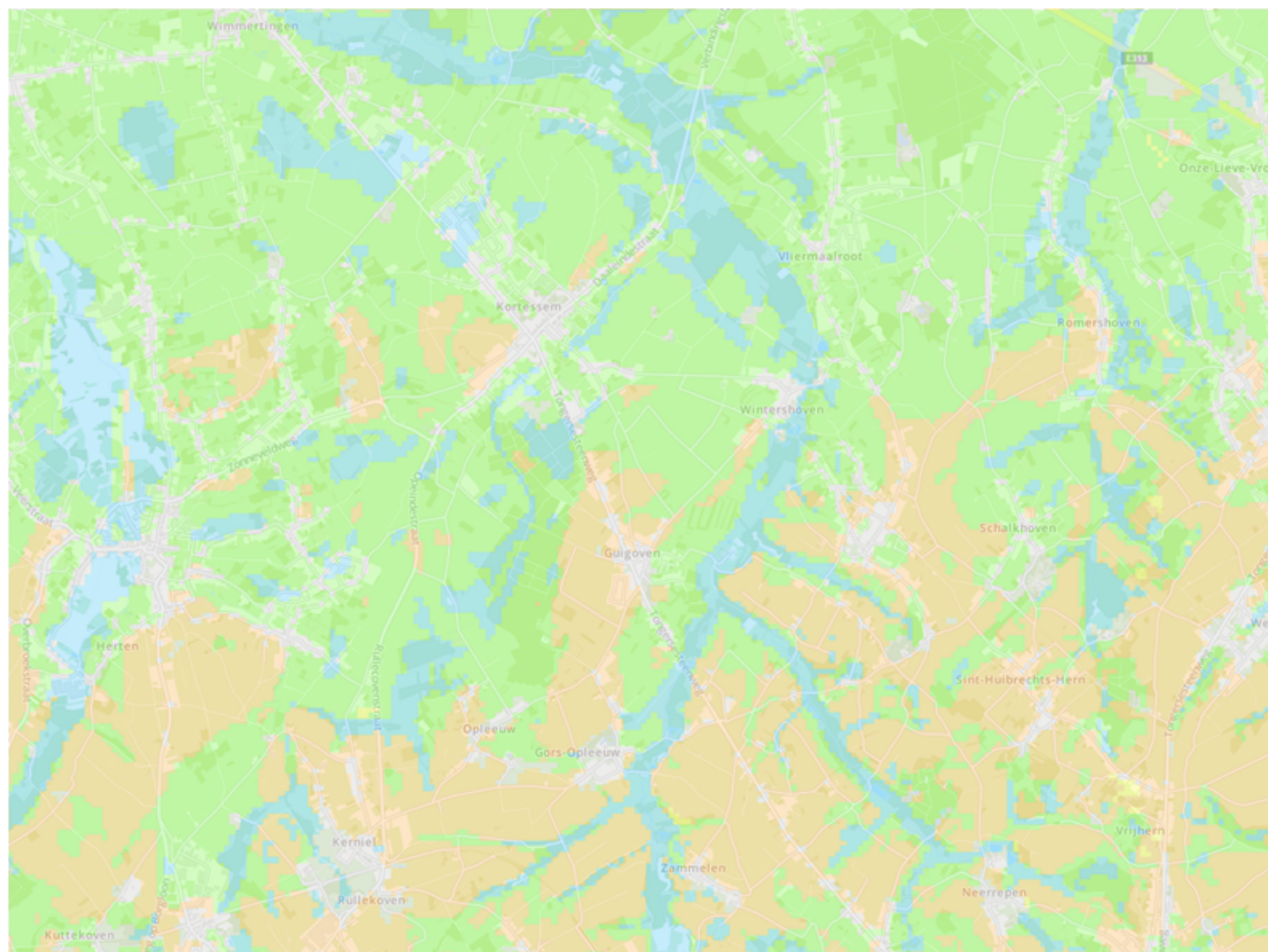
Figuur 25 | Droogtegevoeligheid bodem in Kortessem (huidig klimaat)
