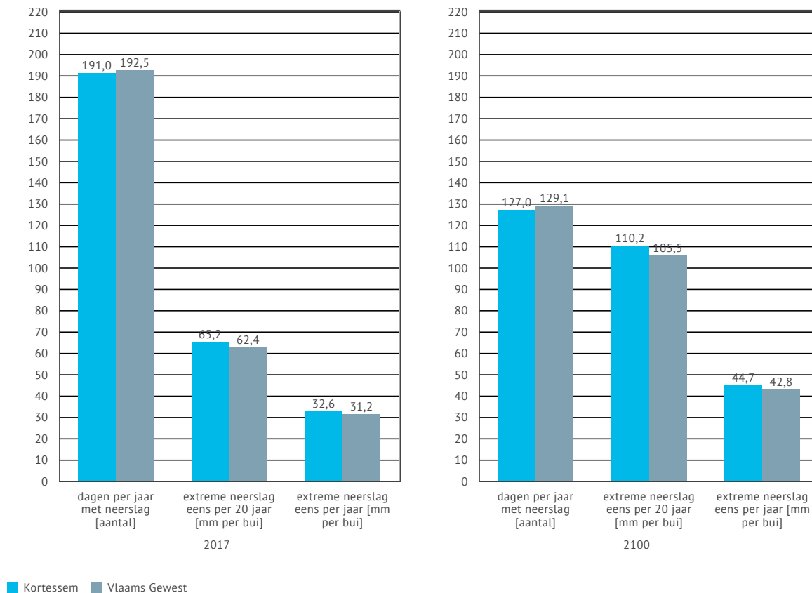
Figuur 12 | Evolutie van (extreme) neerslag in Kortesseem (huidig klimaat en 2100)
