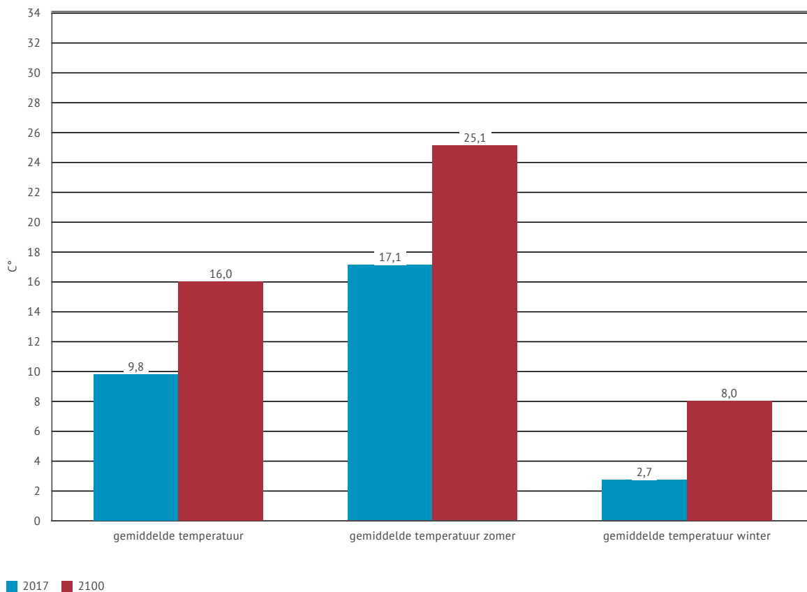
Figuur 32 | Gemiddelde temperatuur in Kortesseem (huidig klimaat en 2100)
