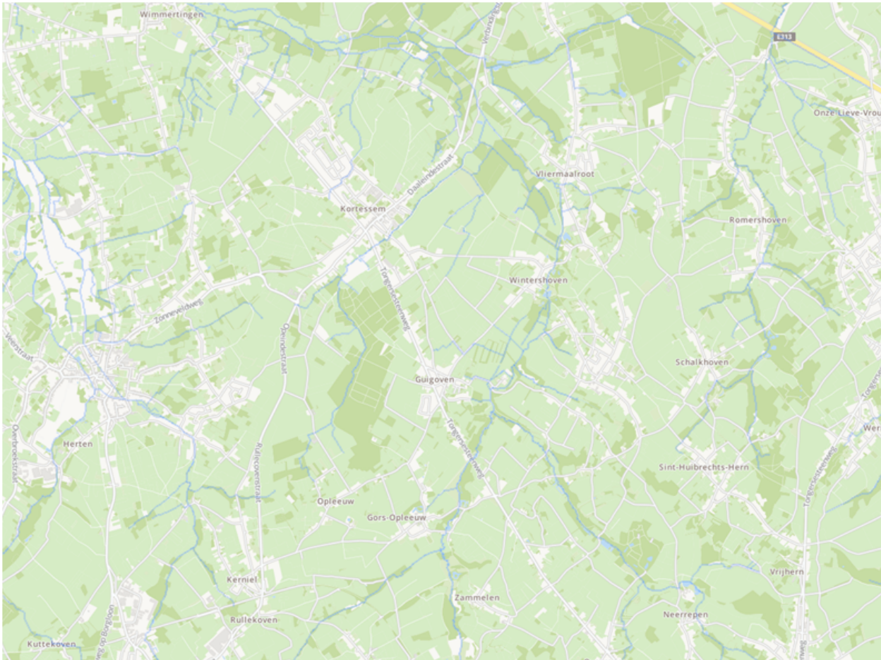
Figuur 13 | Waterlopen in Kortesse
