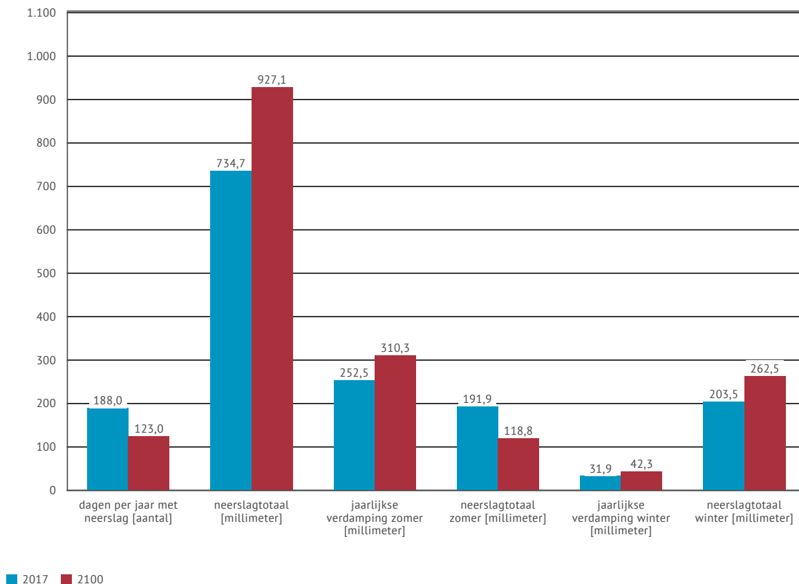
Figuur 24 | Evolutie van de (totale) neerslag en potentiële verdamping in Kinrooi (huidig klimaat en 2100)
