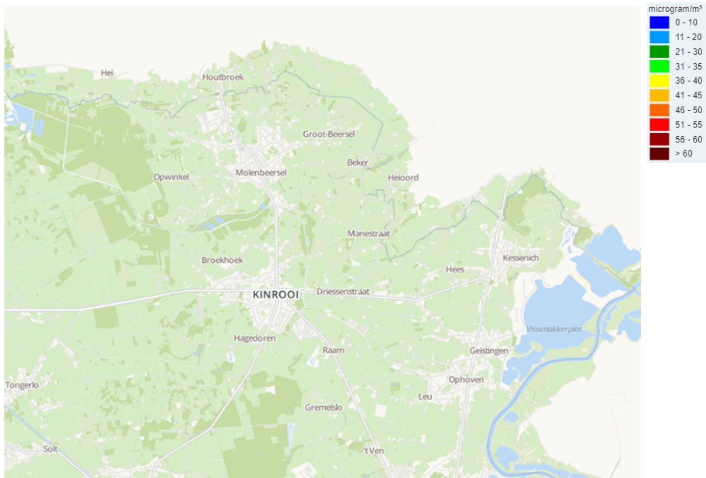
Figuur 09 | Jaargemiddelde ozon (microgram/m 3 ) in Kinrooi (2017)
