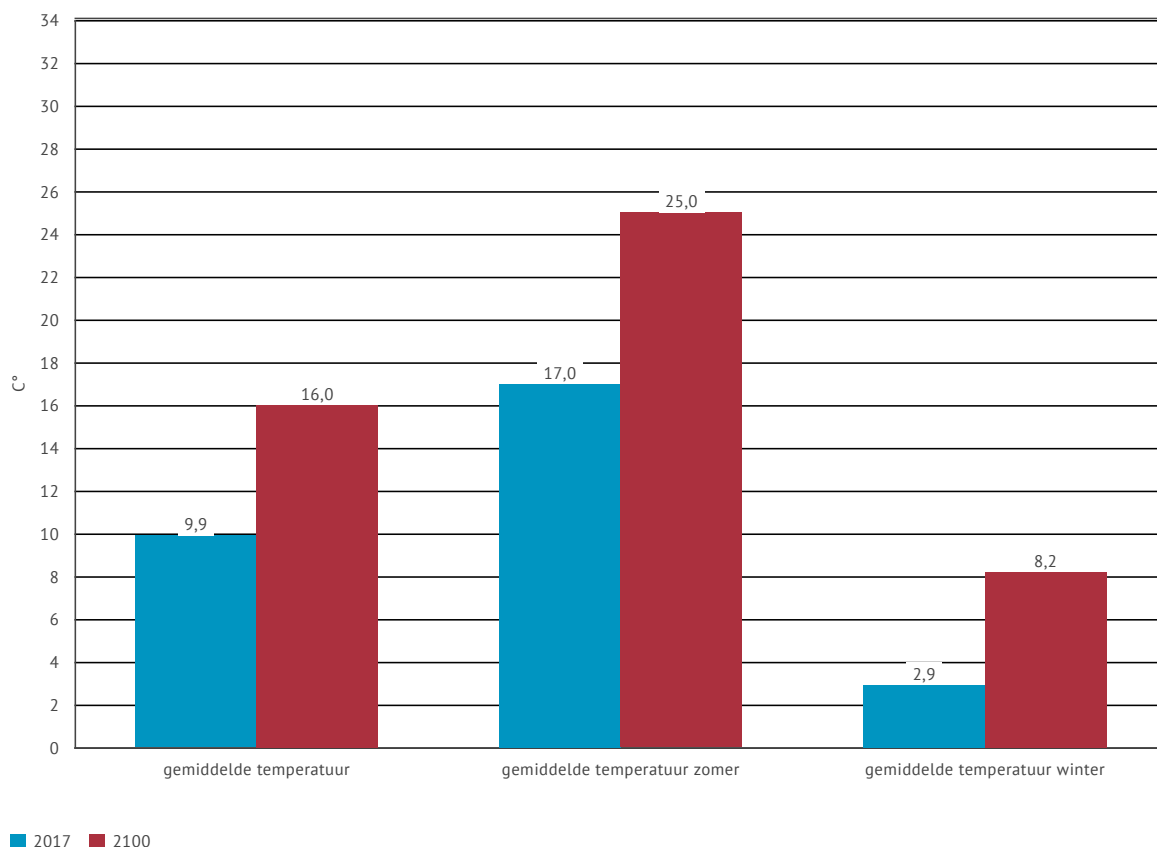
Figuur 32 | Gemiddelde temperatuur in Kinrooi (huidig klimaat en 2100)
