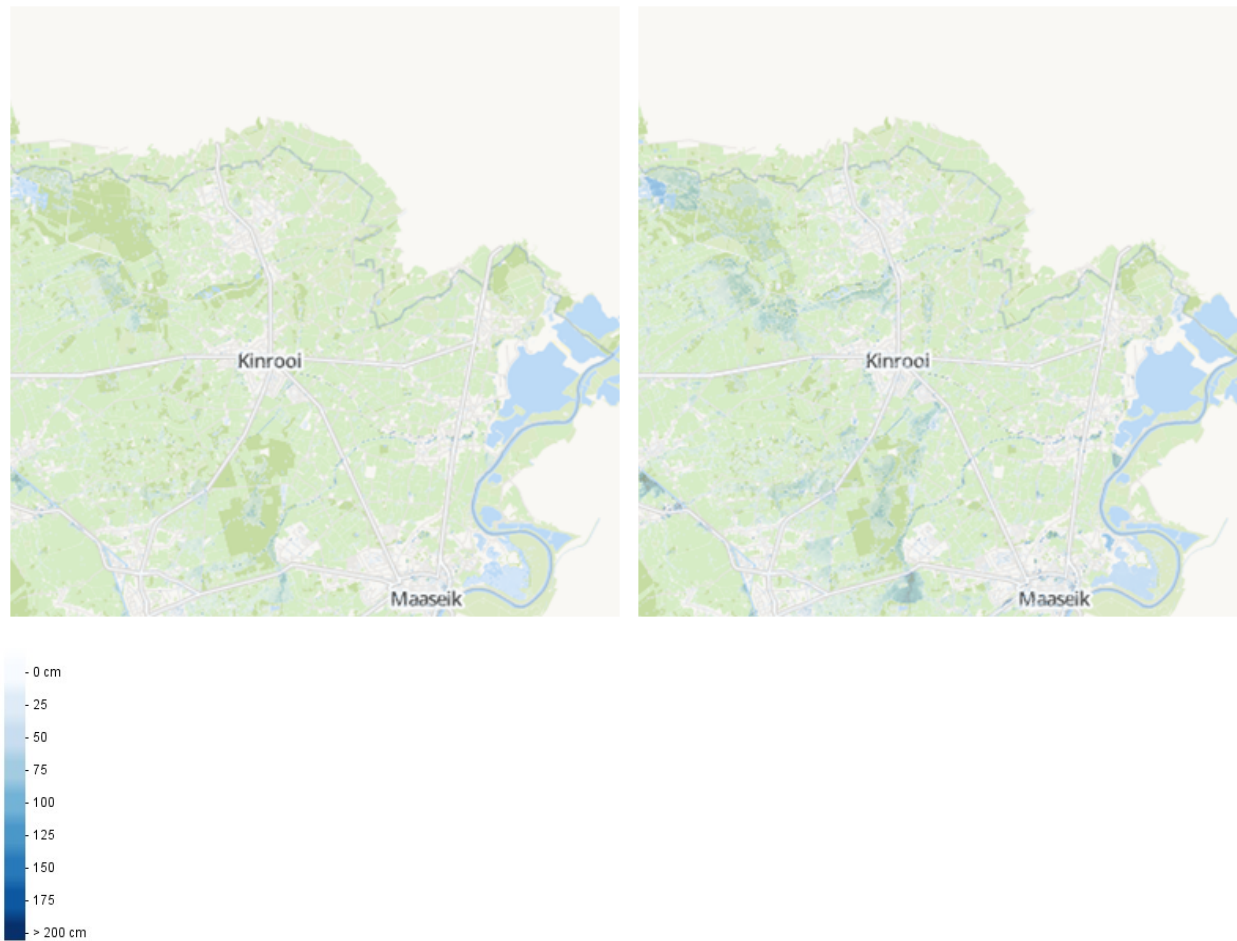
Figuur 17 | Waterdiepte in Kinrooi, in cm (huidig klimaat en 2100)
