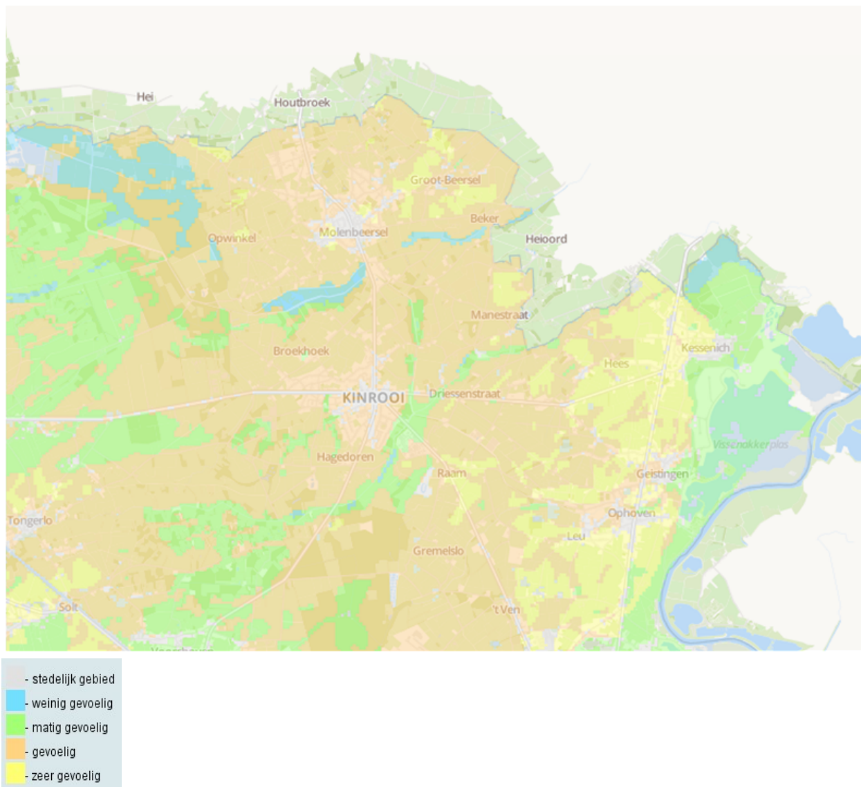
Figuur 25 | Droogtegevoeligheid bodem in Kinrooi (huidig klimaat)
