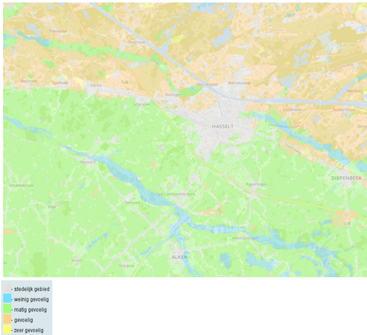
Figuur 25 | Droogtegevoeligheid bodem in Hasselt (huidig klimaat)
