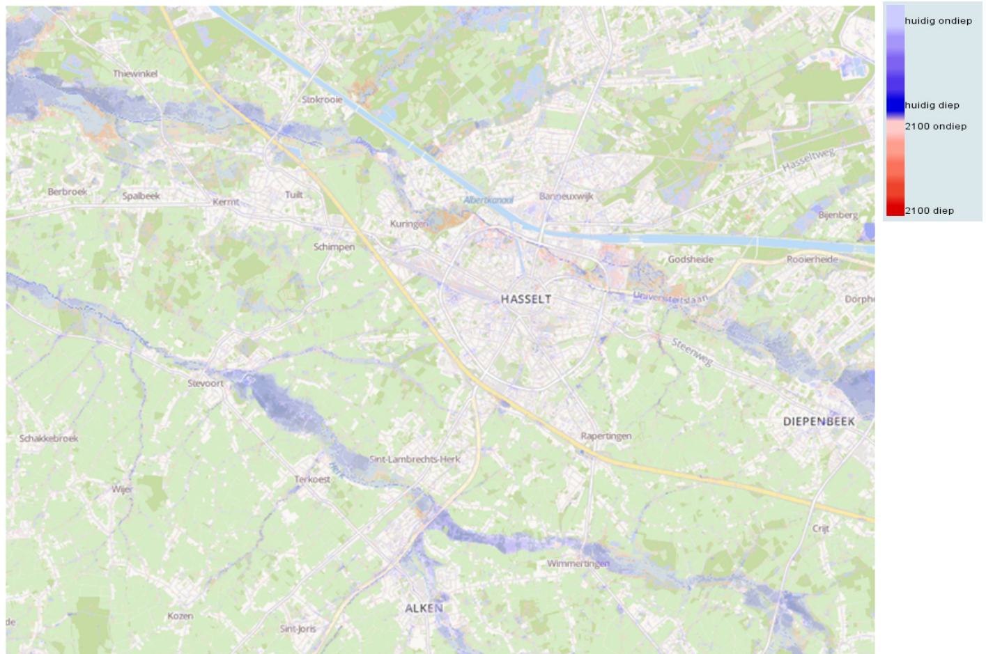
Figuur 18 | Aangroei overstroombaar gebied in Hasselt (2100)
