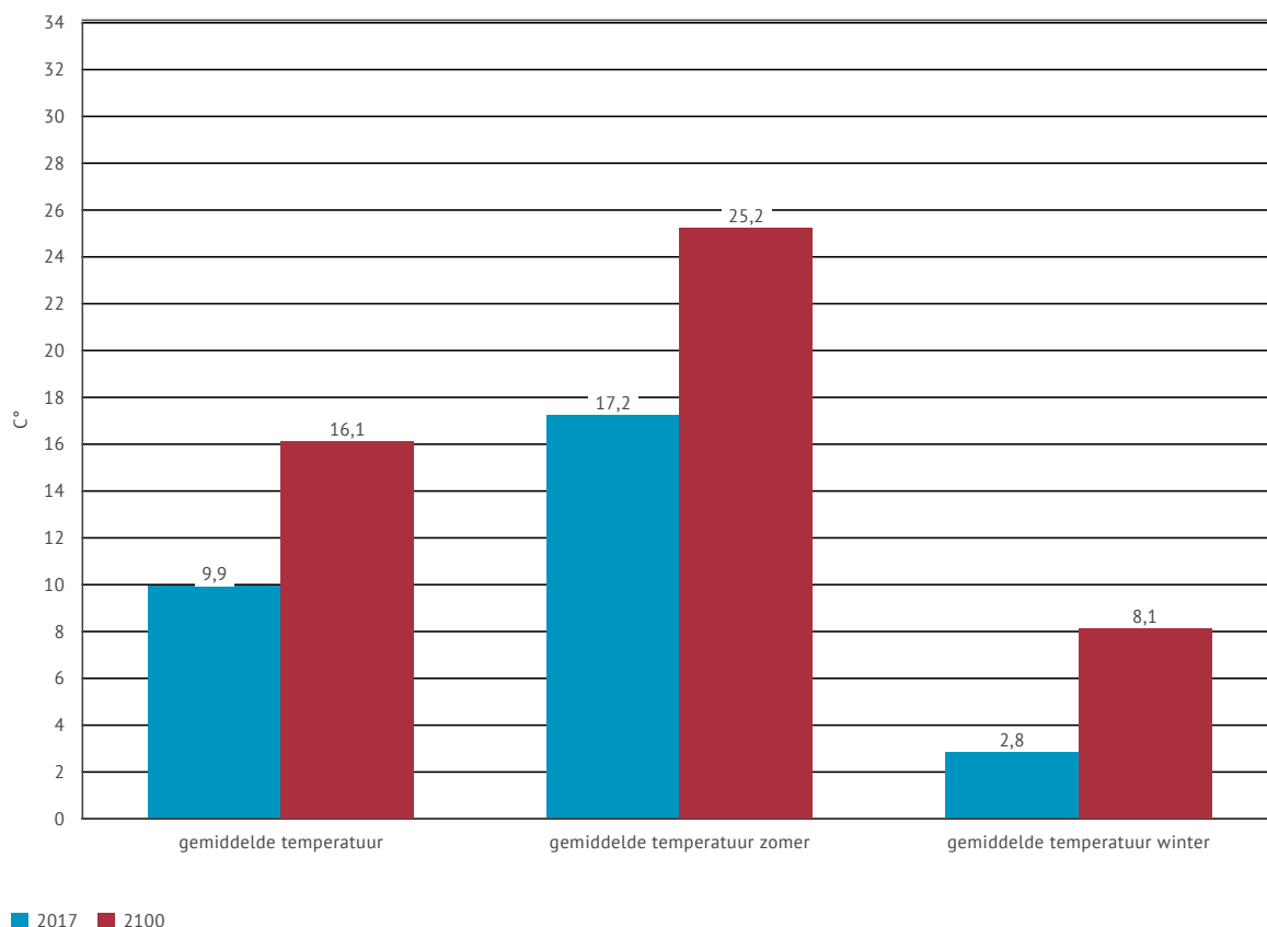
Figuur 32 | Gemiddelde temperatuur in Hasselt (huidig klimaat en 2100)
