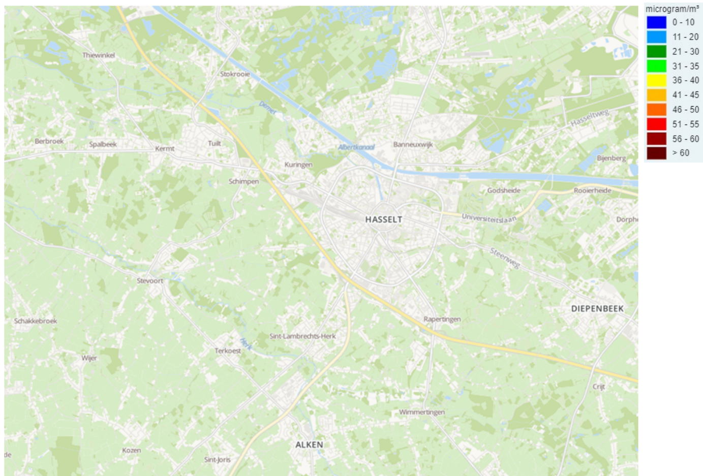
Figuur 09 | Jaargemiddelde ozon (microgram/m 3 ) in Hasselt (2017)
