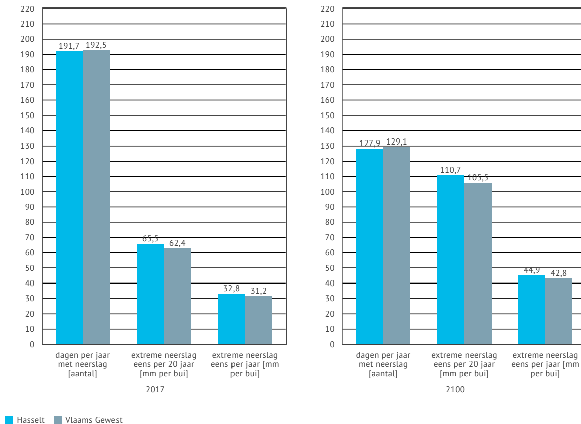
Figuur 12 | Evolutie van (extreme) neerslag in Hasselt (huidig klimaat en 2100)
