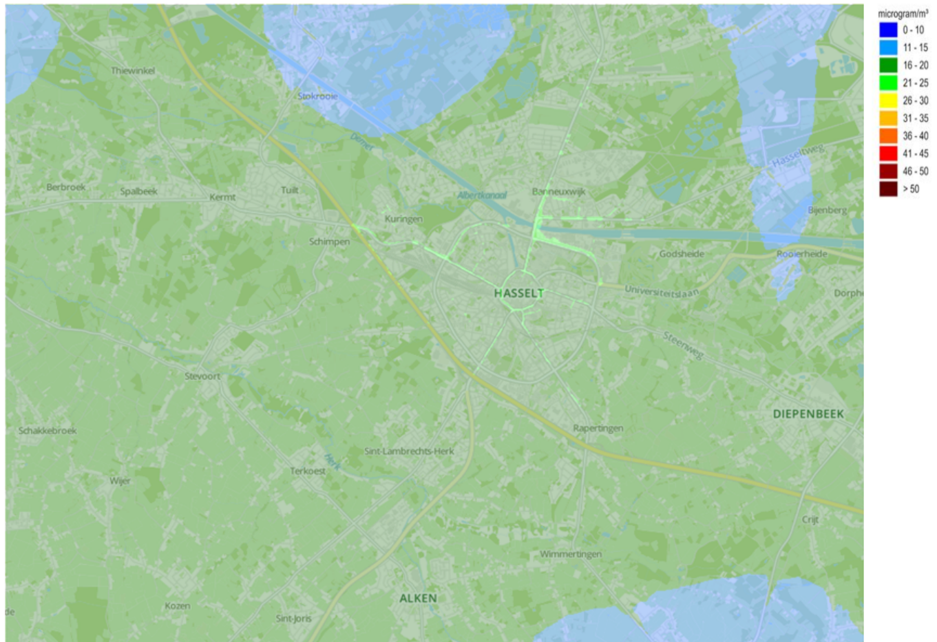
Figuur 42 | Fijn stof in Hasselt (2017)
