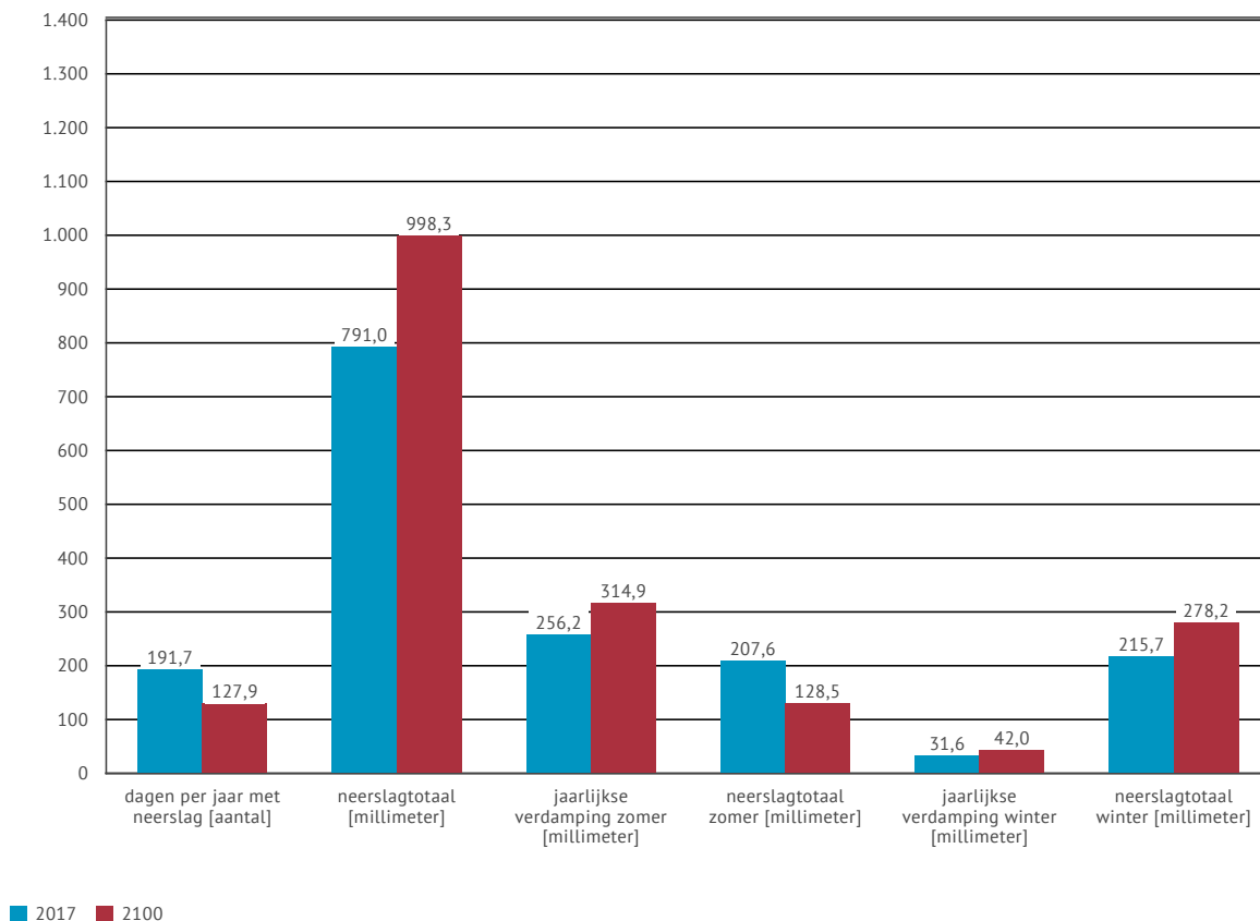
Figuur 24 | Evolutie van de (totale) neerslag en potentiële verdamping in Hasselt (huidig klimaat en 2100)
