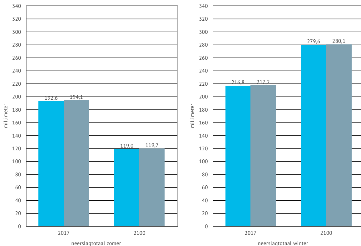
Figuur 11 | Evolutie van het neerslagtotaal in de zomer en in de winter, in mm (huidig klimaat en 2100)
