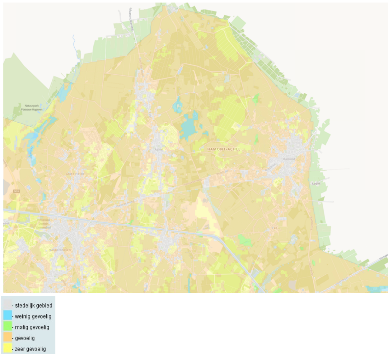
Figuur 25 | Droogtegevoeligheid bodem in Hamont-Achel (huidig klimaat)
