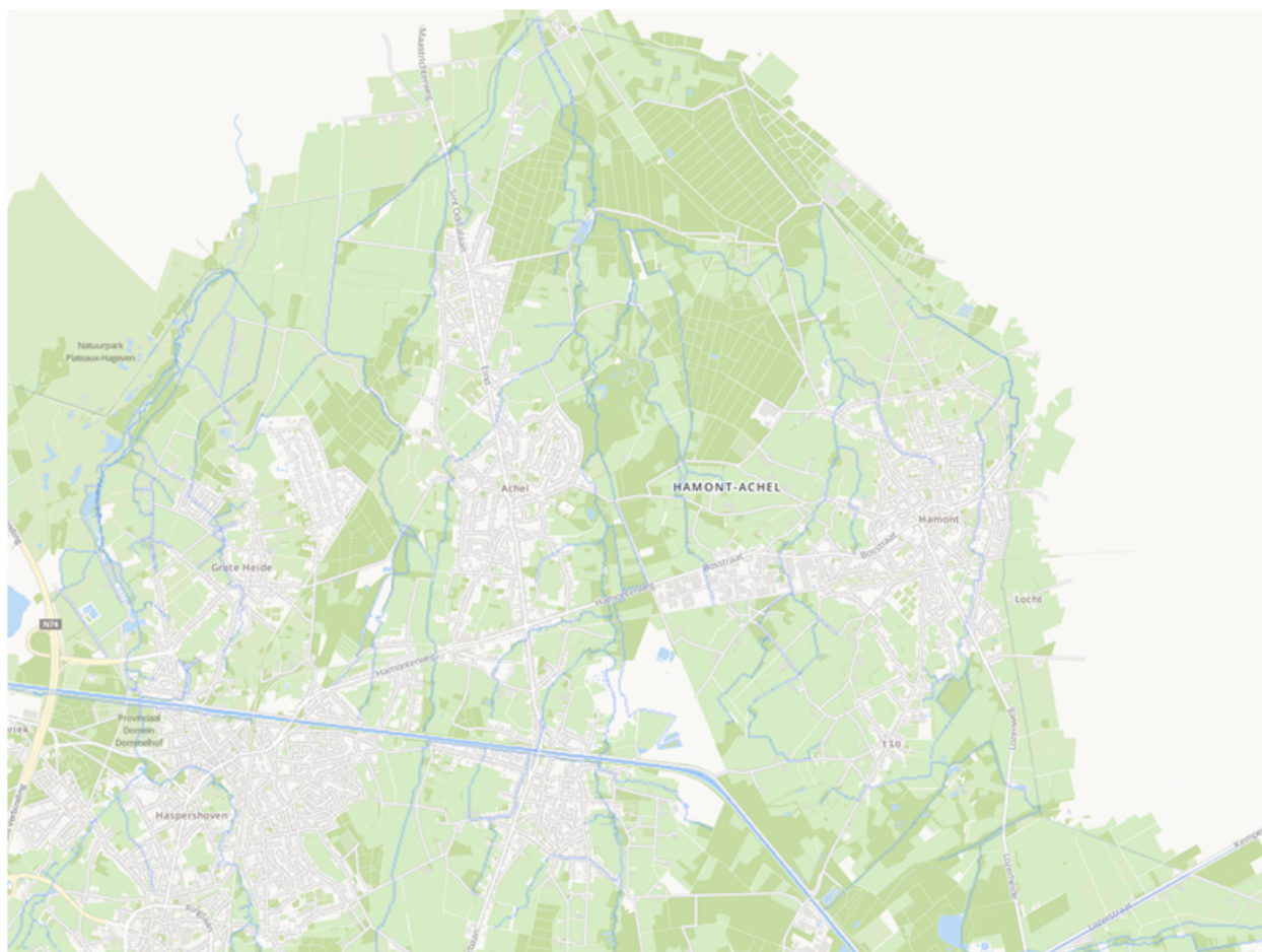
Figuur 13 | Waterlopen in Hamont-Achel
