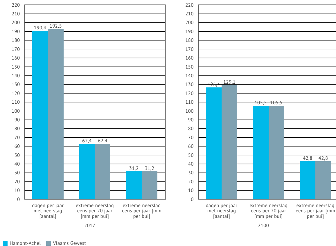
Figuur 12 | Evolutie van (extreme) neerslag in Hamont-Achel (huidig klimaat en 2100)
