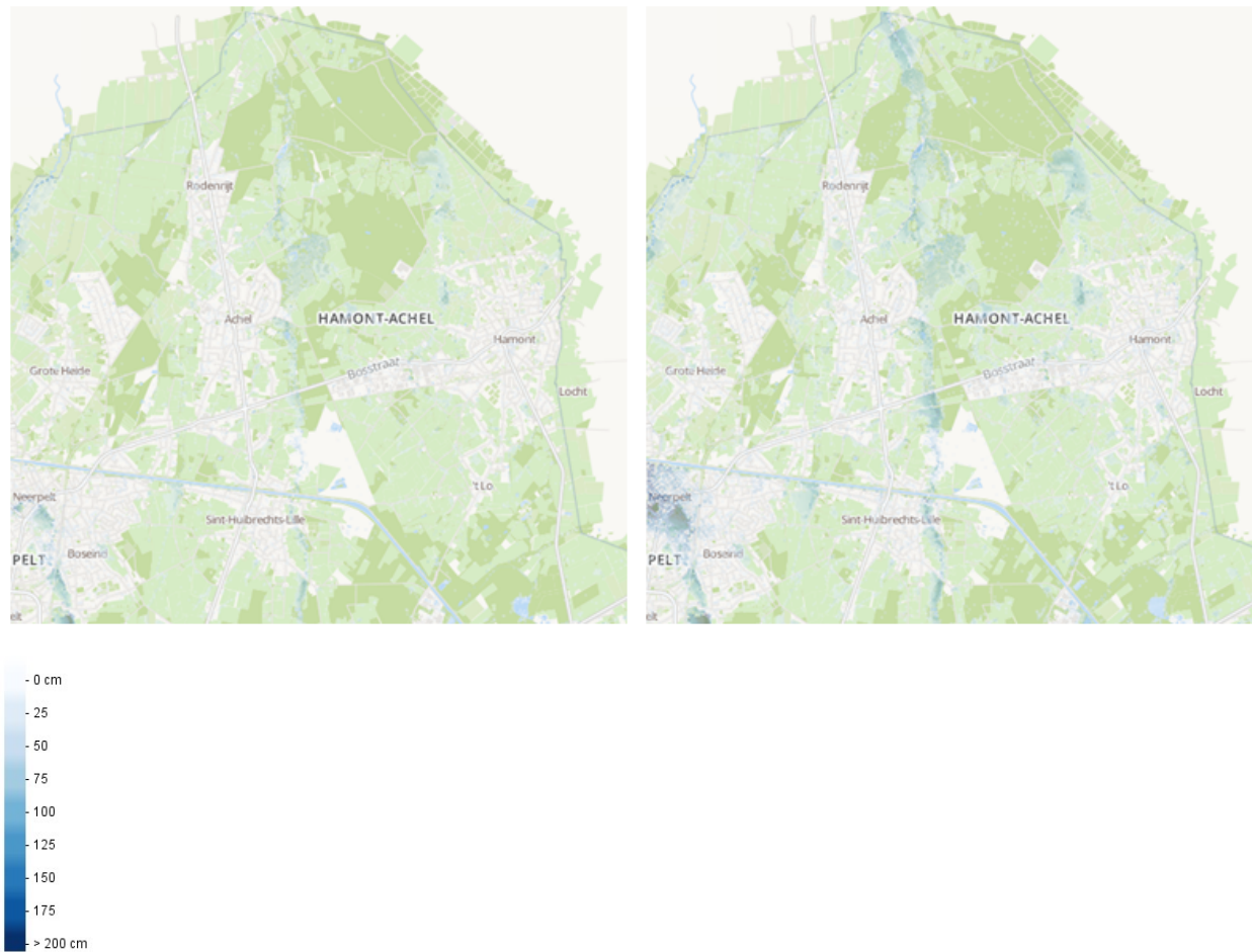
Figuur 17 | Waterdiepte in Hamont-Achel, in cm (huidig klimaat en 2100)
