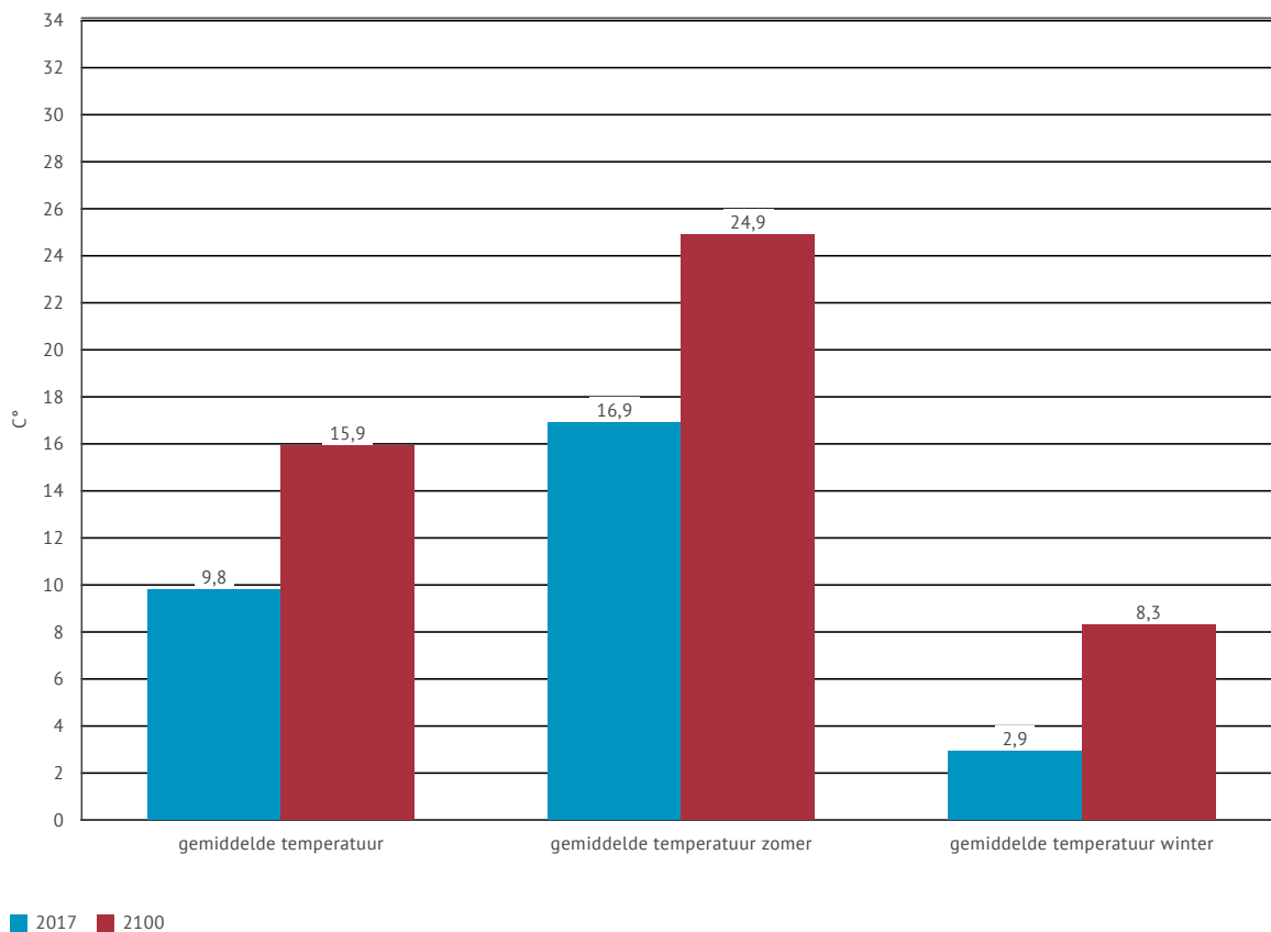
Figuur 32 | Gemiddelde temperatuur in Hamont-Achel (huidig klimaat en 2100)
