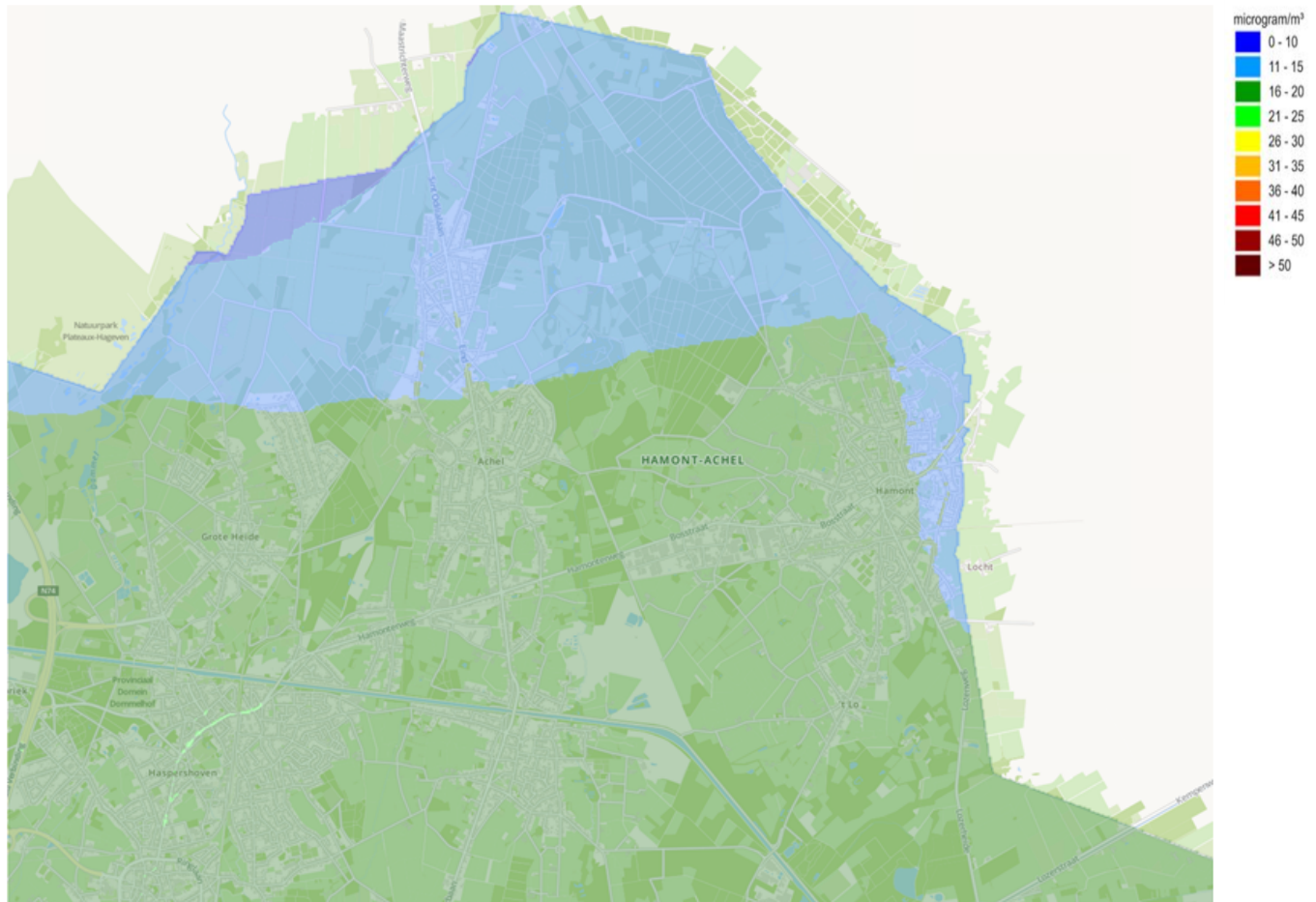
Figuur 42 | Fijn stof in Hamont-Achel (2017)
