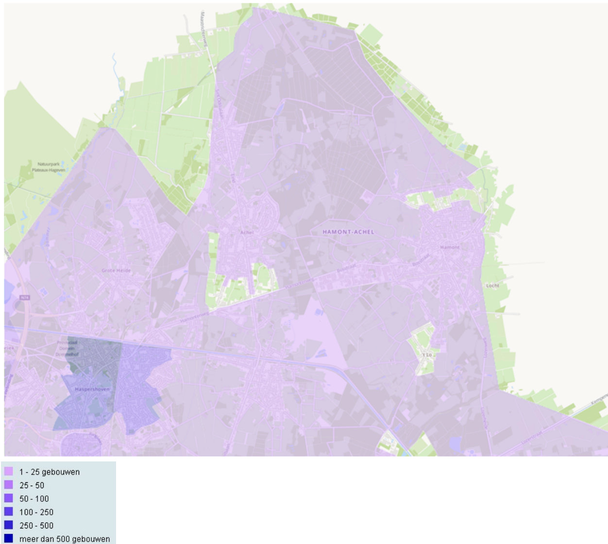
Figuur 22 | Aantal gevaarlijk overstroombare gebouwen in Hamont-Achel (2100)
