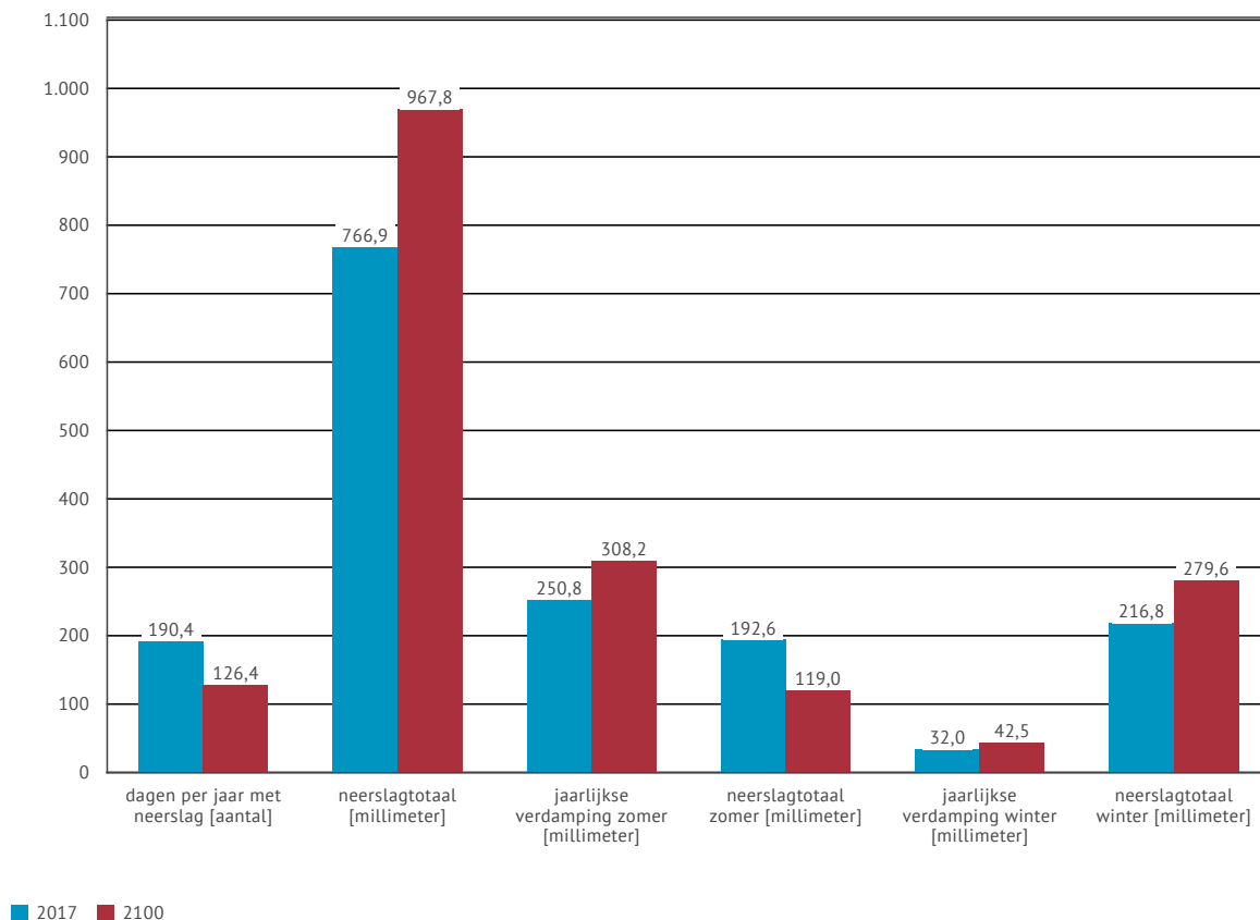
Figuur 24 | Evolutie van de (totale) neerslag en potentiële verdamping in Hamont-Achel (huidig klimaat en 2100)
