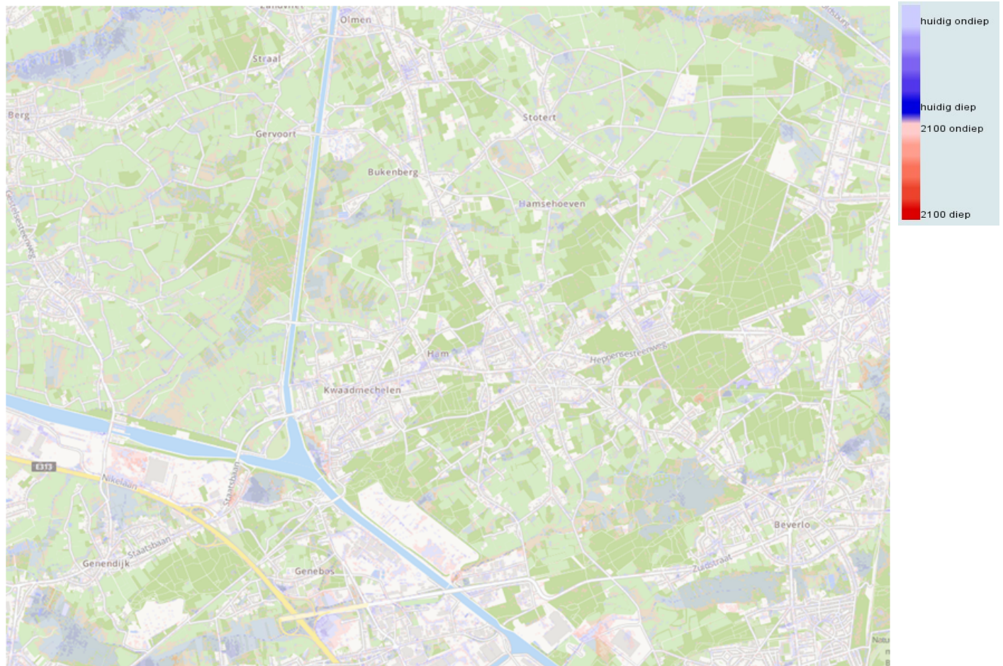
Figuur 18 | Aangroei overstroombaar gebied in Ham (2100)
