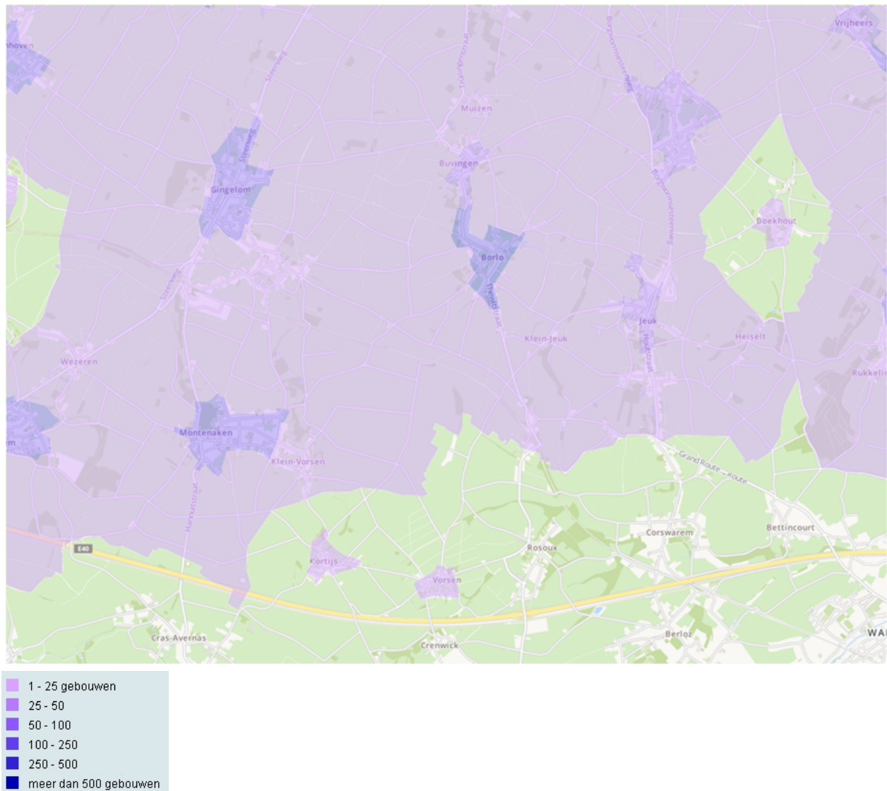
Figuur 22 | Aantal gevaarlijk overstroombare gebouwen in Gingelom (2100)
