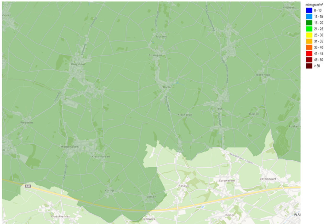
Figuur 42 | Fijn stof in Gingelom (2017)
