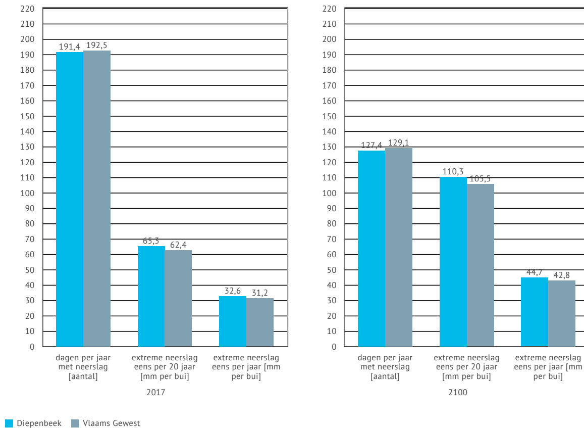
Figuur 12 | Evolutie van (extreme) neerslag in Diepenbeek (huidig klimaat en 2100)
