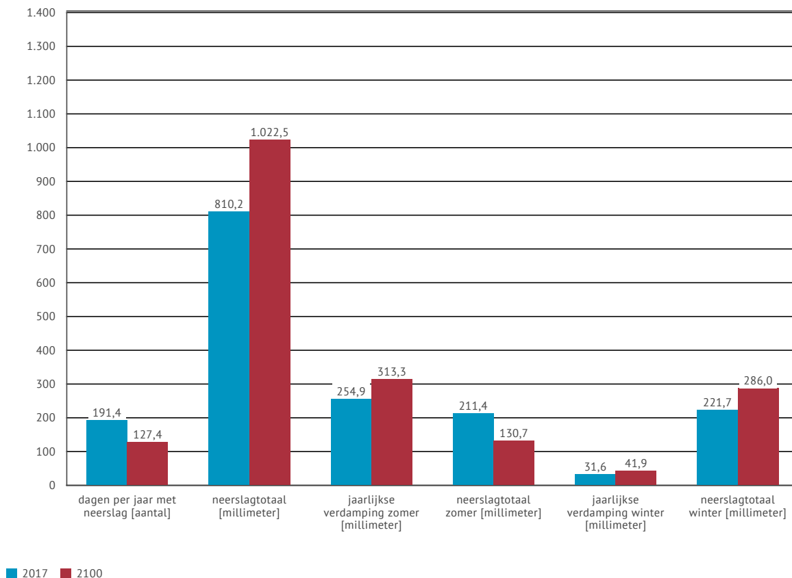
Figuur 24 | Evolutie van de (totale) neerslag en potentiële verdamping in Diepenbeek (huidig klimaat en 2100)
