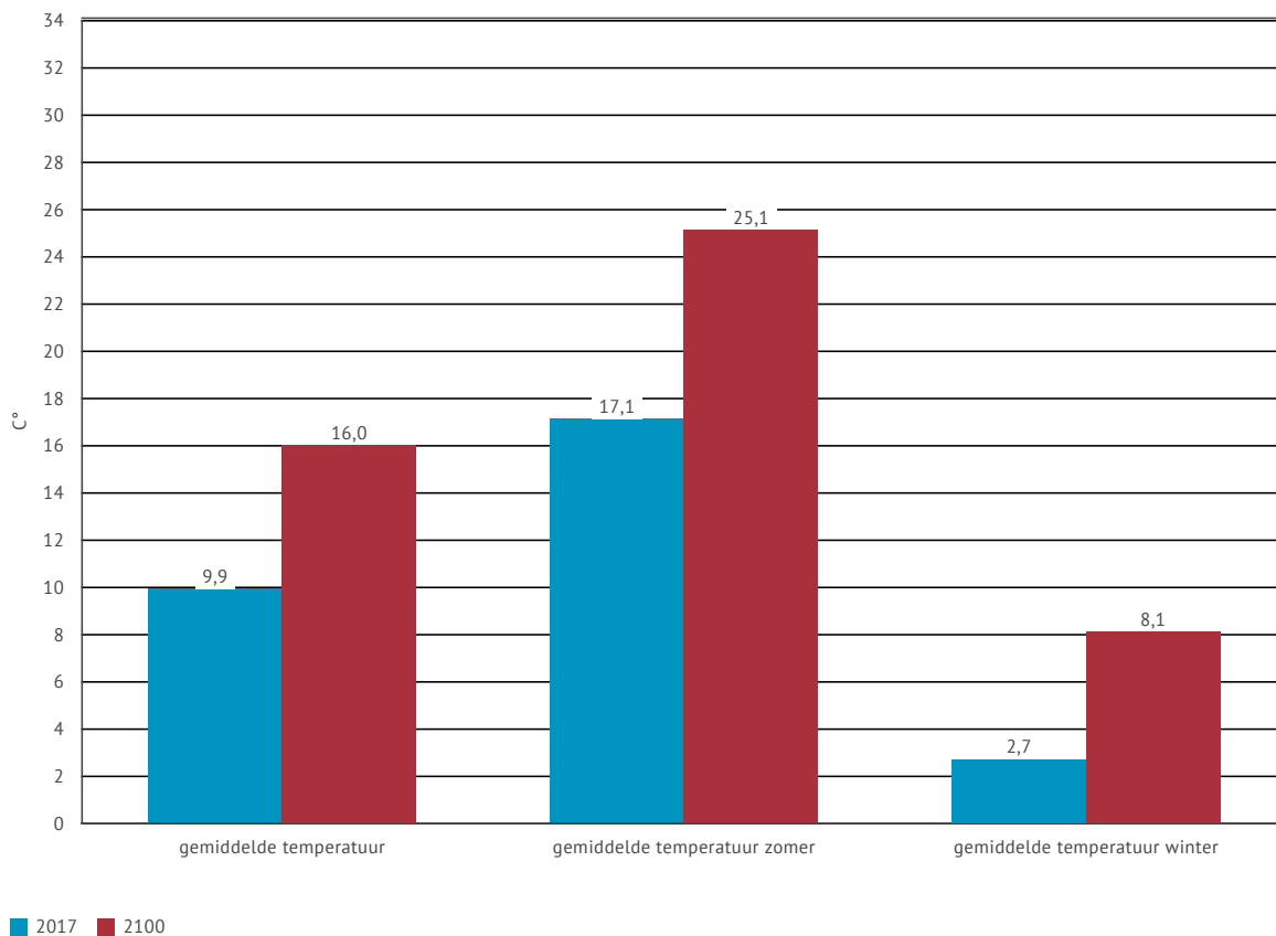
Figuur 32 | Gemiddelde temperatuur in Diepenbeek (huidig klimaat en 2100)
