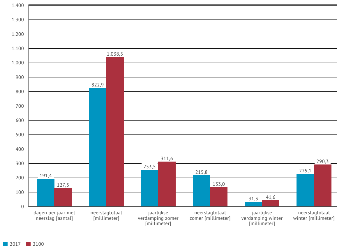
Figuur 24 | Evolutie van de (totale) neerslag en potentiële verdamping in Bilzen (huidig klimaat en 2100)
