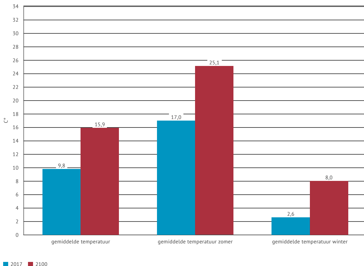
Figuur 32 | Gemiddelde temperatuur in Bilzen (huidig klimaat en 2100)
