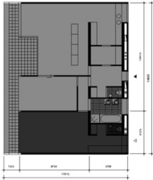
BASIS-TYPE 3 kamerappartementen
